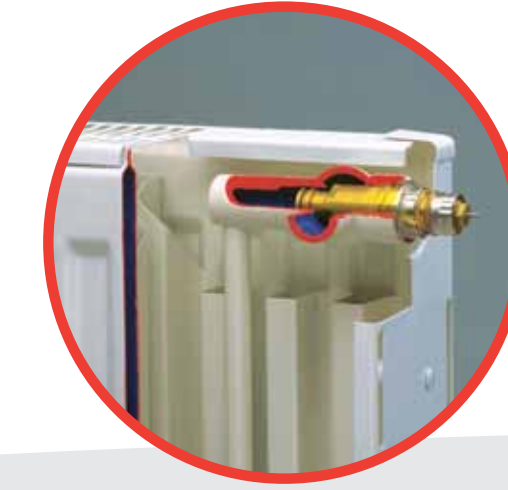
Kompakt Termostatik Radyatör Çekirdeği
